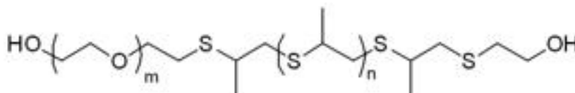
PPS-PEG
